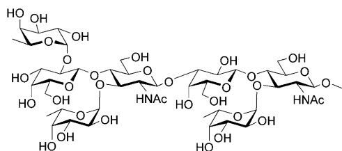
Figure 1. Le y Le x heptasaccharide.
